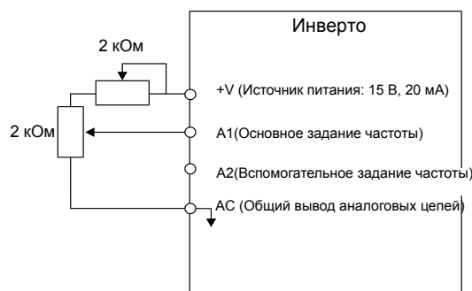
Рис. 6.6 Поддача основного задания частоты
