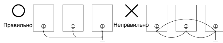
Рис. 2.9 Подключение заземления
