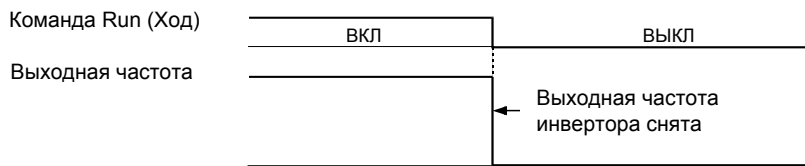
Рис. 6.15 Остановка с вращением по инерции
